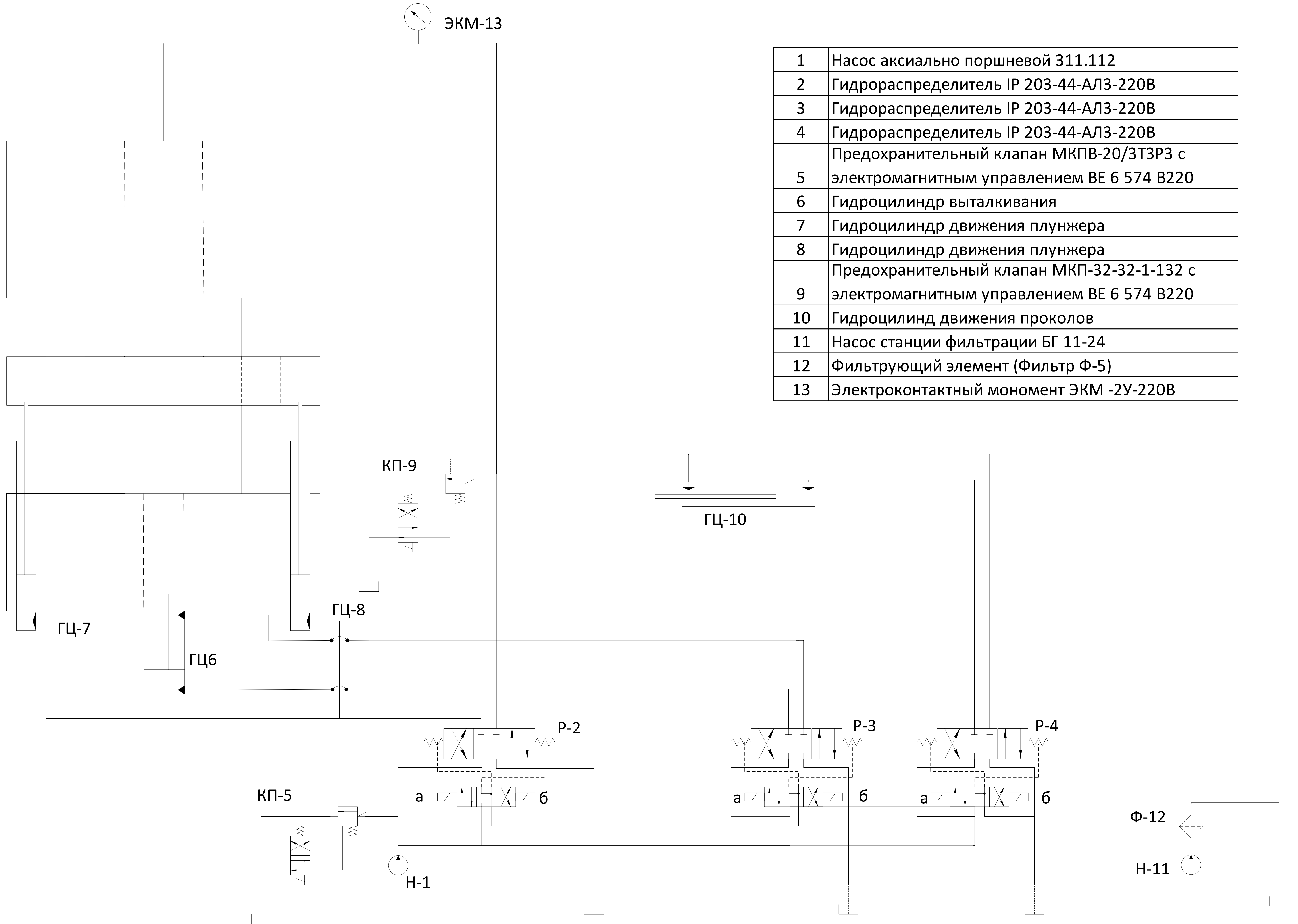
Схема гидравлическая пресса П-457
